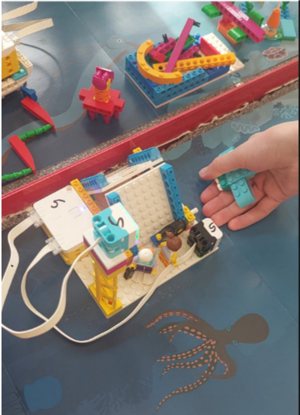
Fisch-Zählstation Fische unterschiedlicher Farben werden gezählt (mit Farbsensor).
